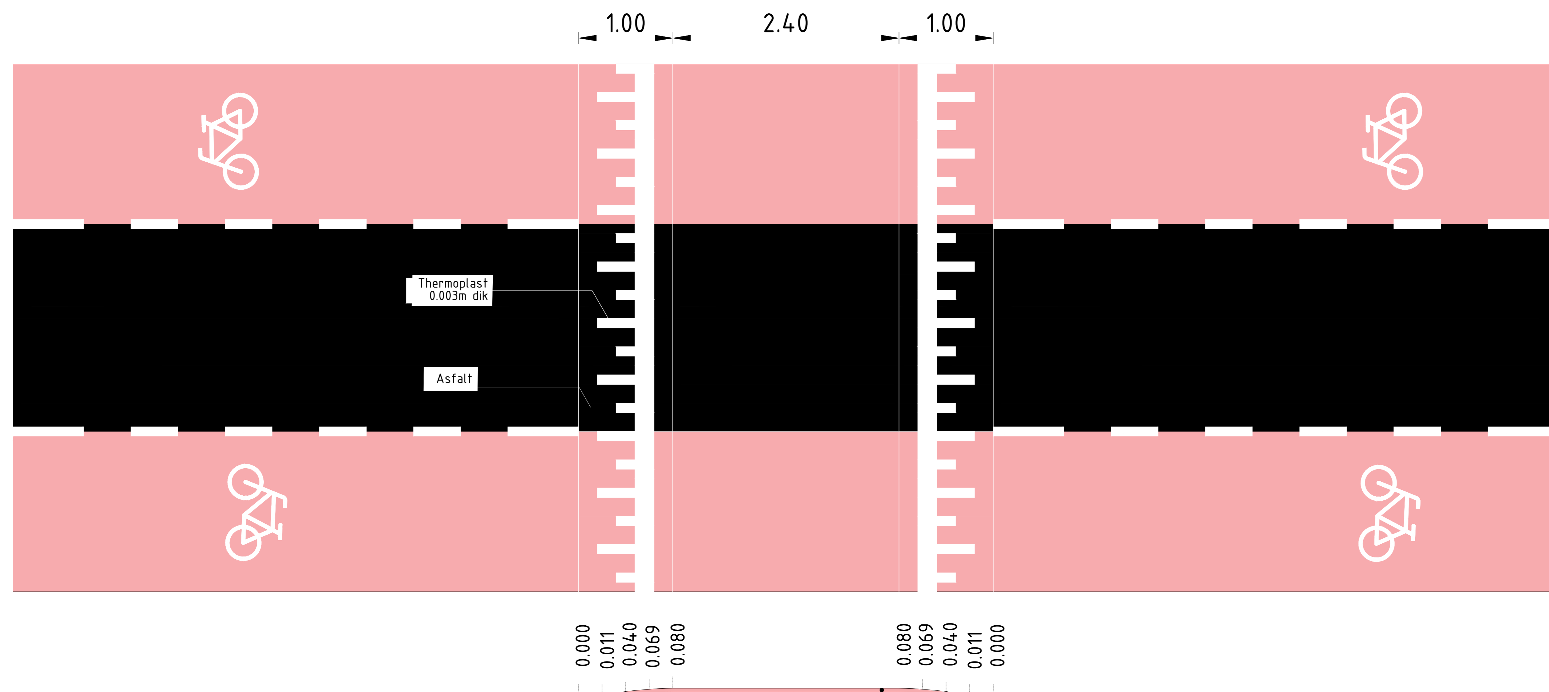
Detail sinusdrempel 30km/u Schaal 1:50
