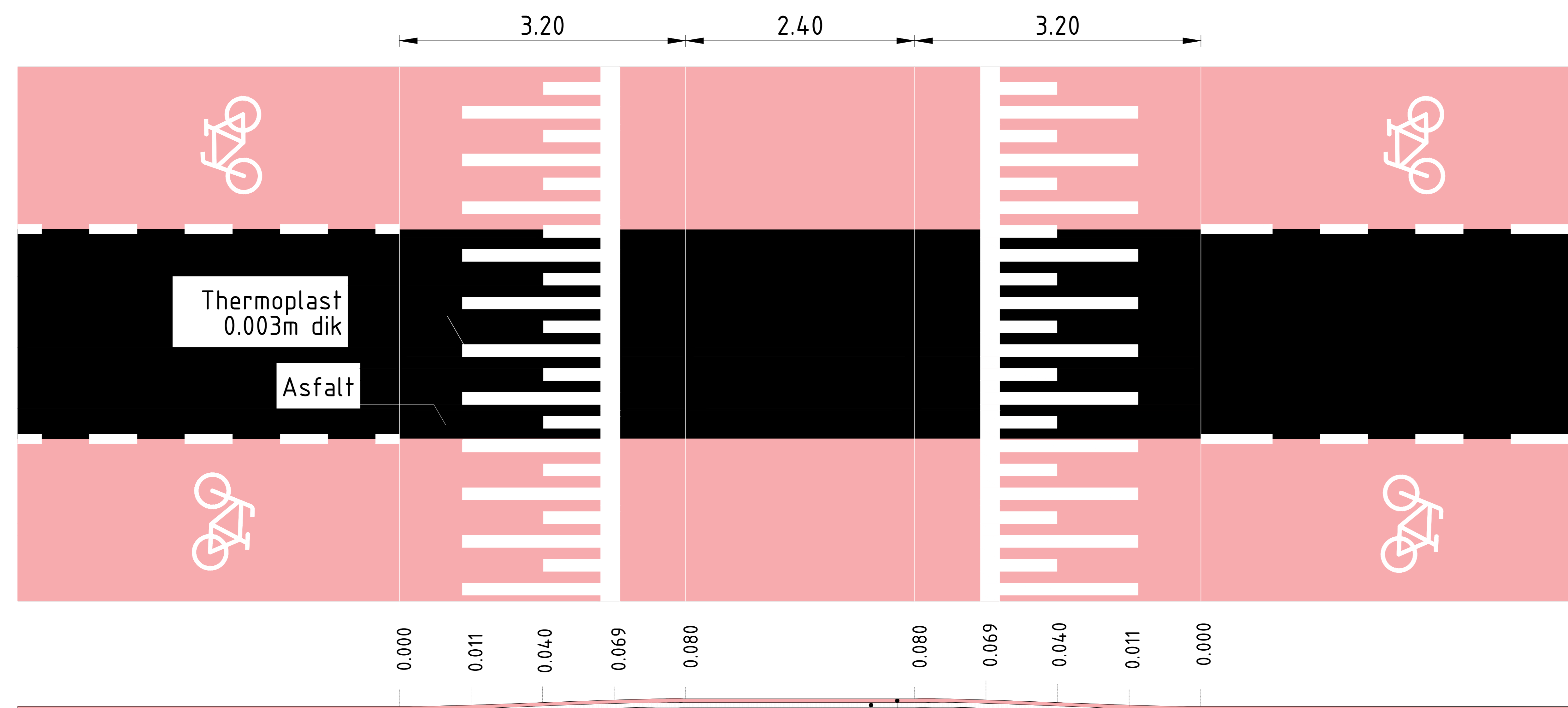
Detail sinusdrempel 60km/u Schaal 1:50
