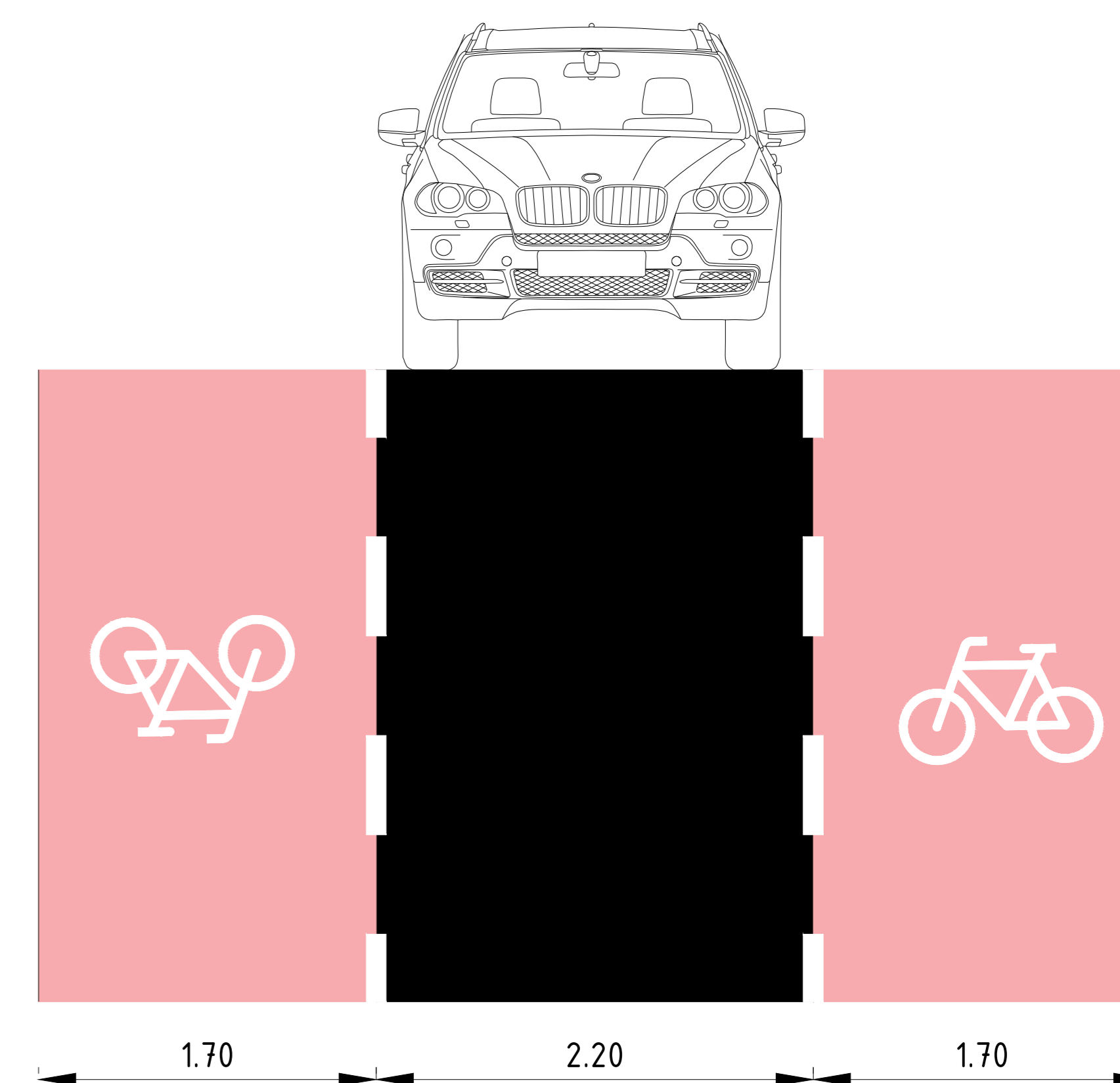
Doorsnede rijbaan/fietspad Schaal 1:50
